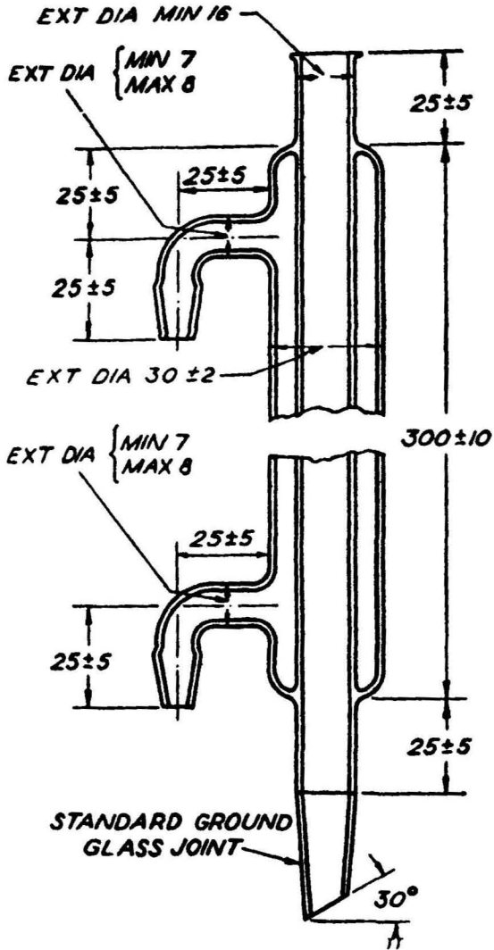
FIG. 2 CONDENSER
