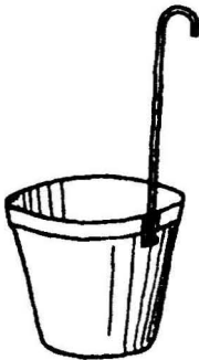
FIG. 1 BITUMEN SAMPLER
